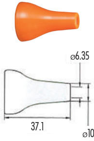
Buse droite Ø6.35 mm
