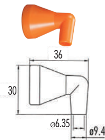
Buse coudée à 90° Ø9.5 mm
