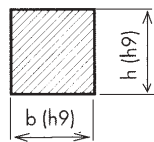
Section carrée
