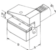
Type B3 : court inversé à droite
