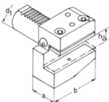
Type B2 : court à gauche
