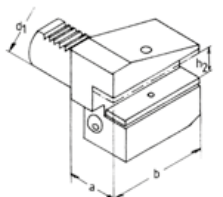
Type B4 : court inversé à gauche
